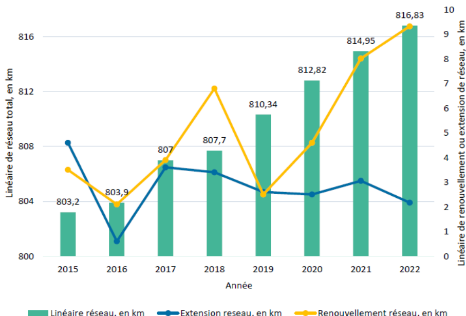
Evolution du réseau de distribution d'eau potable depuis 2015
